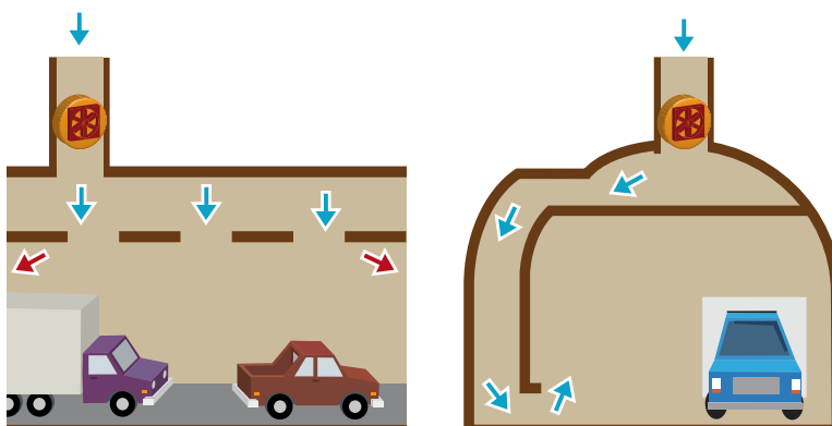
Semi-Transverse Ventilation
