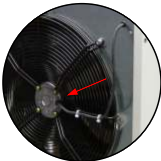
Вентилатор със самосмазващи се лагери, вградена термична защита и дебит до 8950 m 3 /h
